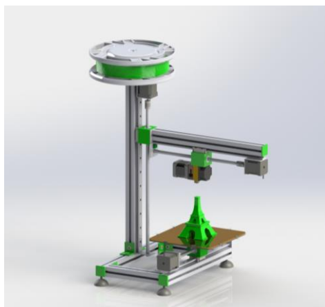
Machine 3D à dépôt de fil fondu.
